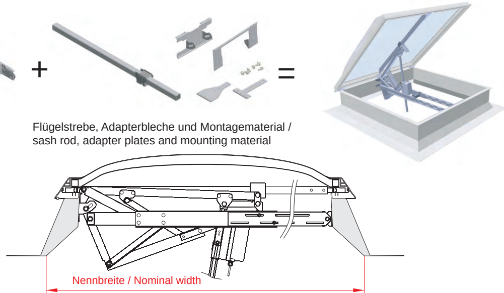
Grundmodul inkl. Antrieb / basic module incl. drive
